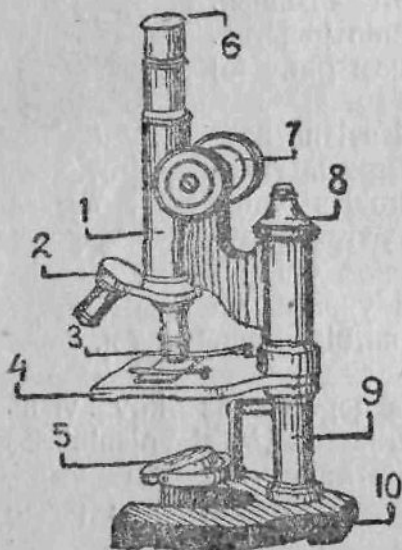
68-d şerpas. 1. Trubka. 2. Revolver. 3. Obyektiv. 4. Pəzan. 5. Zerkala. 6. Okular. 7. Pina ıvəd vint. 8. İcət mikrometriçeskə vint. 9. Stativ. 10. Kok.
